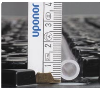
Systémová doska Minitec o hrúbke 1 cm
