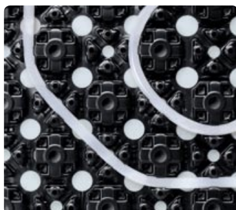
Rúrky možno inštalovať aj v 45° uhle
