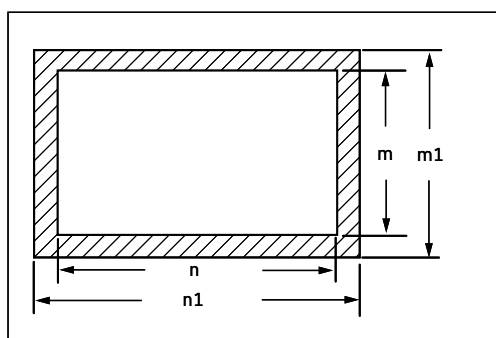
Rozměry výřezu Starck K
