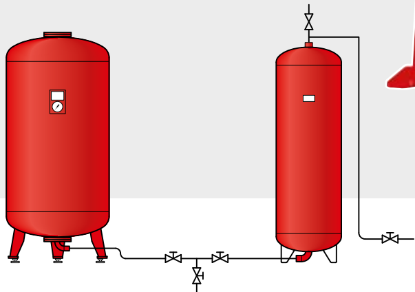
Pripojovacia schéma predradenej nádoby Flexcon
