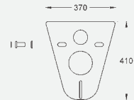
2x 37 131 000 Odhlučňovací set pro WC , 2 gumová pouzdra
