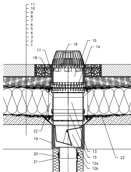
ZATEPLENÁ STŘECHA – ZATRAVNĚNÍ EXTENZIVNÍ, KLASICKÉ POŘADÍ VRSTEV HYDROIZOLACE Z ASF. PÁSŮ
