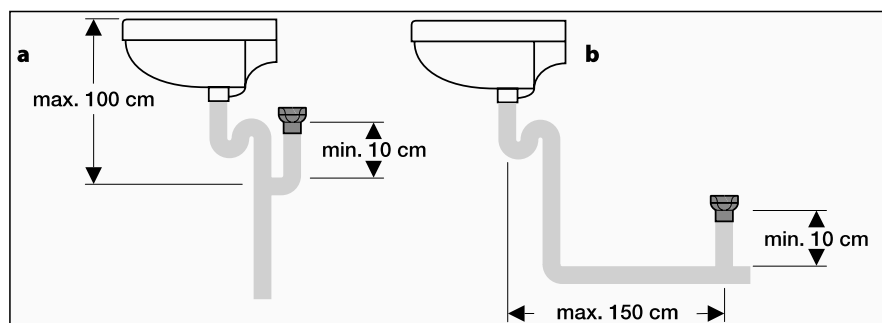
Obr. 1 Prívzdušňovací ventil u umyvadla a – na svislé části pripojovacího potrubí; b – na ležaté části pripojovacího potrubí
