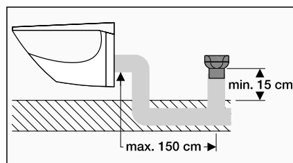
Obr. 3 Prívzdušňovací ventil pro WC na ležatém pripojovacím potrubí
