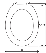
rozmery v mm: A 410-450 B 360 C 425
