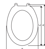
rozmery: A 440-470 mm B 370 mm C 440 mm
