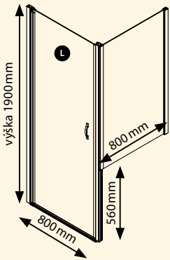
Skleněná výplň
