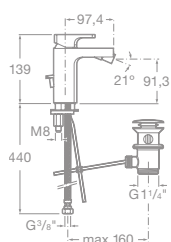
75A6301C00 Bidetová stojančeková batéria s bočnou pákou, s automatickou zátkou, chróm, 315,57 €
