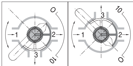
Obr. 9 - zapojení jako rozdělovací armatura
