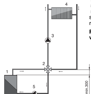
Obr. 2 - Příklad zapojení směšovače Duomix do systému
