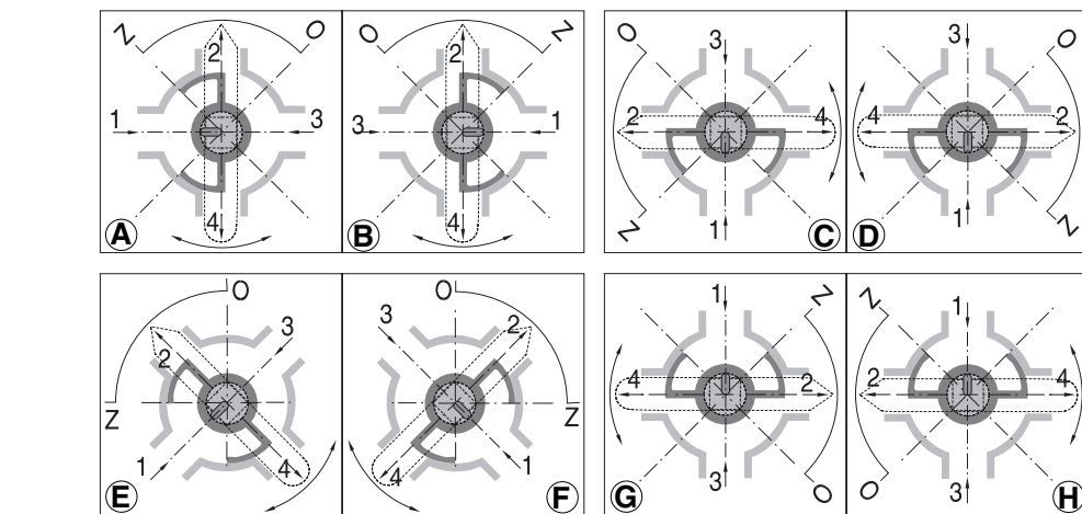
Obr. 7 - Možnosti zapojení směšovačů Duomix
