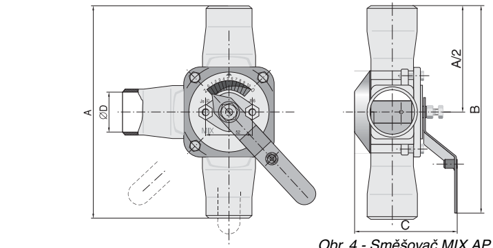
Obr. 4 - Směšovač MIX AP
