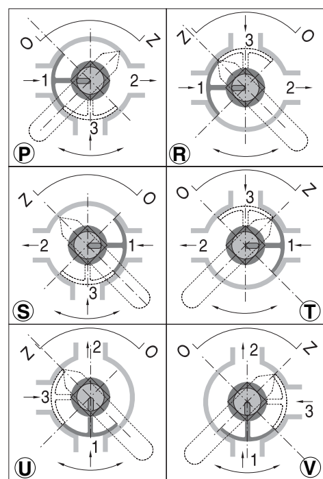
Obr. 8 - Možnosti zapojení směšovačů MIX
