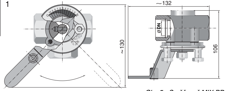
Obr. 5 - Směšovač MIX BP
