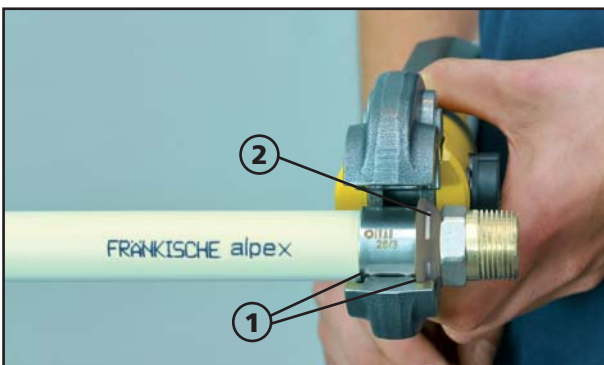
Správne založenie vodiaceho plastového krúžku tvarovky do fixačnej drážky čeluste typu „B“
