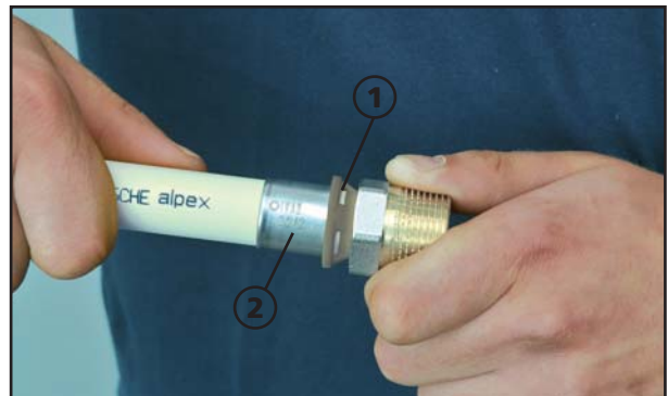
Detail správneho zasunutia tvarovky IVAR.PRESS na potrubie IVAR.ALPEX:
