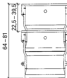
Rozsah nastavenia s nadstavcom s odrezanými upevňovacími okami
