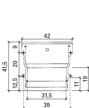
Rozsah nastavenia s nadstavcom s upevňovacími okami
