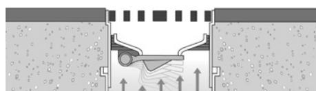
Funkčná schéma spätnej klapky MEASTOP UNIVERSAL
