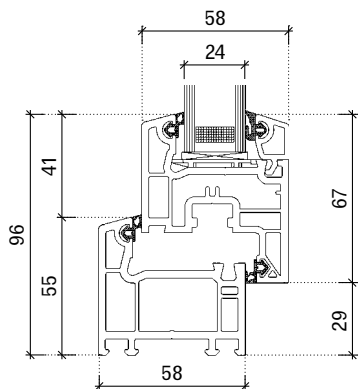
Prierez profilom MEALON otvárávo – sklopné, Standard , šírka rámu 58 mm
