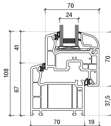
Prierez profilom MEALON otvárávo – sklopné, Komfort , šírka rámu 70 mm
