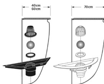
Protizápachový uzáver pre svetlíky s hĺbkou 40/60a 70 cm
