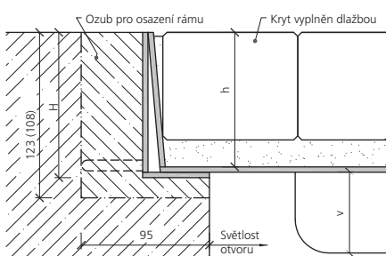
Detail osadenia rámu do stavebného otvoru
