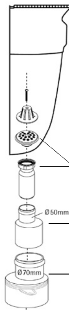
Odvodňovacia prípojka so sitkom
