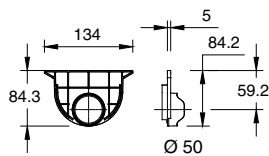
Čelná stena plná s predformovaným odtokom DN50
