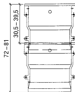
Rozsah nastavenia s nadstavcom s upevňovacími okami
