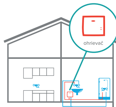
Ilustračný obrázok HAKL MX zapojenie ohrievača do vodovodného systému.
