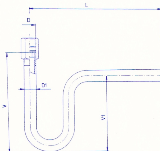
Připojovací a stavební rozměry
