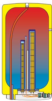
Elektrický zásobník
