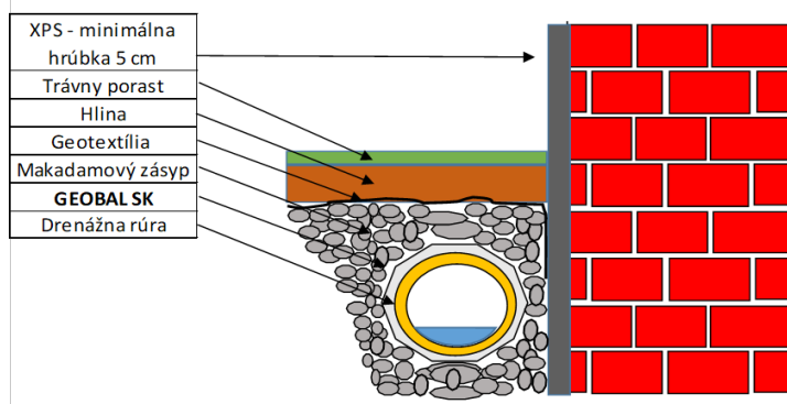
Izolácia základov
