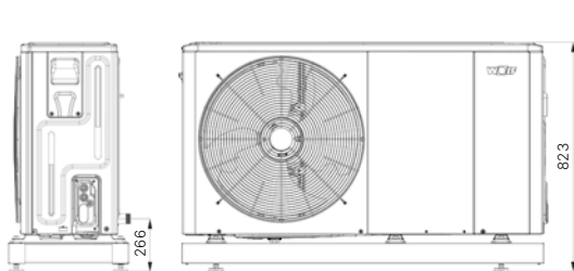
Rozmery vonkajšej jednotky FHA 05/06, 06/07 so základnou konzolou
