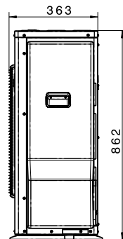
vonkajšia jednotka BWL-1S(B)-05/07
