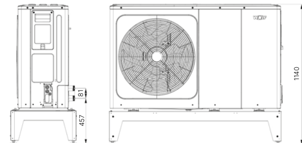
Rozmery vonkajšej jednotky FHA 08/10, 11/14, 14/17 s podlahovou konzolou
