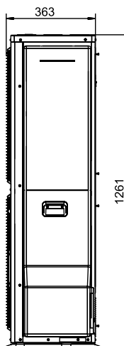
vonkajšia jednotka BWL-1S(B)-10/14/16
