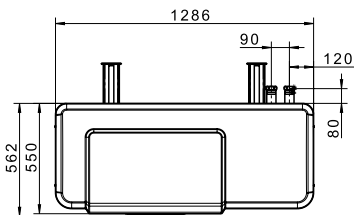
vonkajšia jednotka so stenovou konzolou
