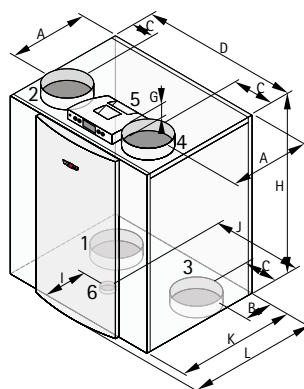
Pripojenie 2/2 L
