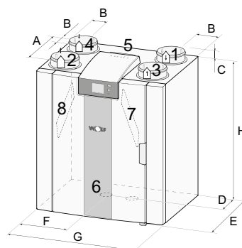
Pripojenie 4/0 R
