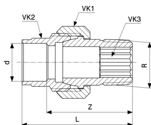
Prechodový skrutkový spoj - červený bronz alebo kremíkový bronz, mosadz model 94341G
