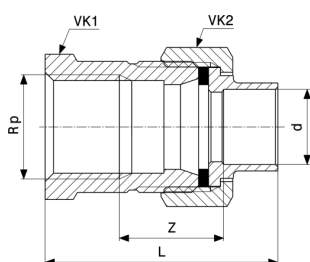
Prechodový skrutkový spoj - červený bronz, mosadz model 94330G
