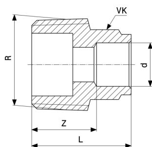
Prechodový kus - červený bronz model 94243G
