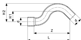
Nadoblúk - meď model 95086
