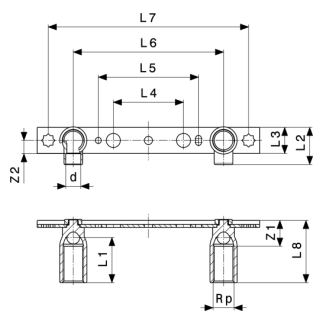
Gemini-montážna jednotka model 94476
