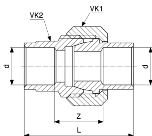
Skrutkový spoj - červený bronz model 94340
