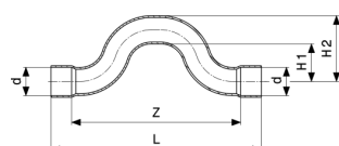
Nadoblúk - meď model 95085
