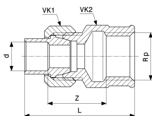
Prechodový skrutkový spoj - červený bronz alebo kremíkový bronz, mosadz model 94340G
