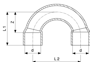
Oblúk 180° - meď model 95060
