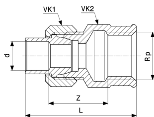
Prechodový skrutkový spoj - červený bronz alebo kremíkový bronz, mosadz model 94340G
