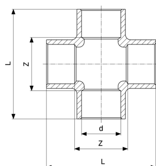
Křížový kus - červený bronz model 94180
