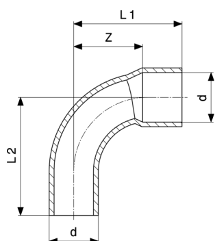
Oblúk 90° - meď model 95001A
