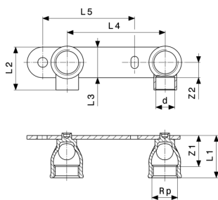
Gemini-montážna jednotka model 94476.2
