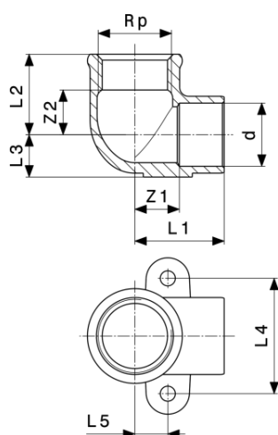
Nástenka - červený bronz model 94472G
