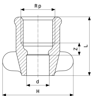
Prechodový kus - červený bronz model 94270GF
