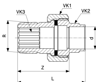
Prechodový skrutkový spoj - červený bronz, mosadz model 94331G
