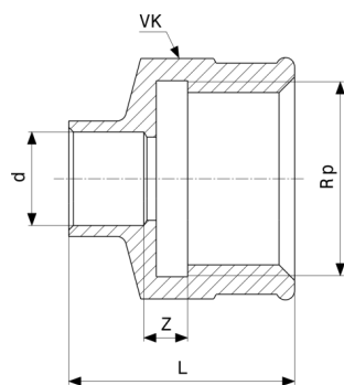
Prechodový kus - červený bronz model 94270G
