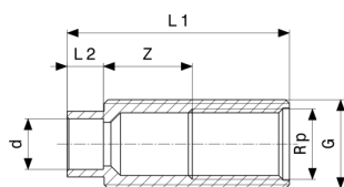
Stenová priechodka - červený bronz model 3427.2
