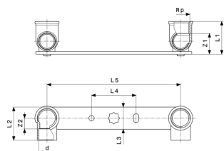
Gemini-montážna jednotka model 94476.0
