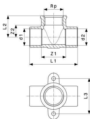
Nástenka T-kus - červený bronz model 94490G
