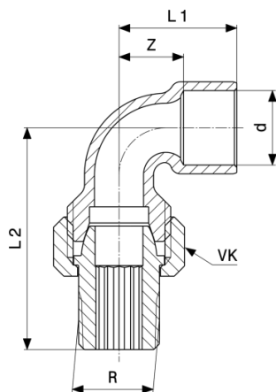
Prechodový skrutkový spoj 90° - červený bronz alebo kremíkový bronz, mosadz model 94098G
