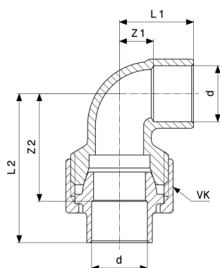
Prechodový skrutkový spoj 90° - červený bronz model 94096
