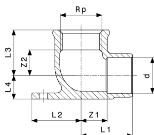
Nástenka - červený bronz model 94471G
