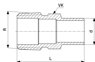
Prechodový kus - červený bronz model 94280G
