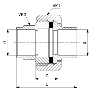
Skrutkový spoj - červený bronz model 94330
