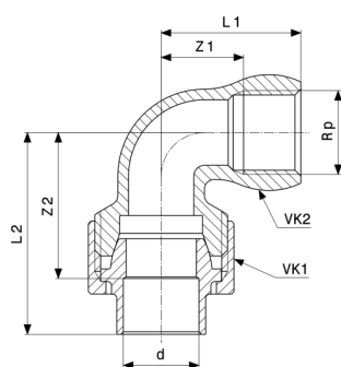
Prechodový skrutkový spoj 90° - červený bronz alebo kremíkový bronz, mosadz model 94096G
