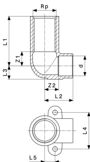
Nástenka - červený bronz model 94472GL
