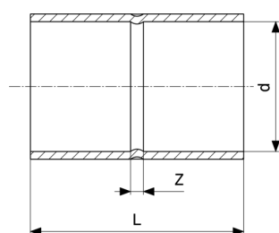
Spojka - meď model 95270
