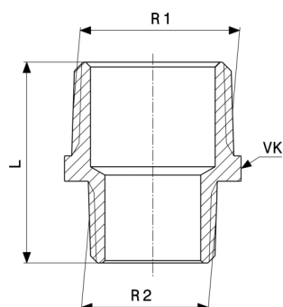
Redukční vsuvka - červený bronz nebo křemíkový bronz model 3245
