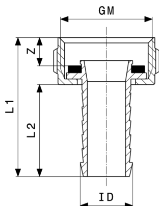
Hadicový skrutkový spoj - mosadz model 1817
