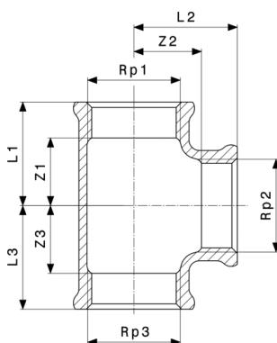
T-kus - červený bronz alebo kremíkový bronz model 3130
