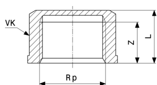
Viečko - červený bronz alebo kremíkový bronz model 3301
