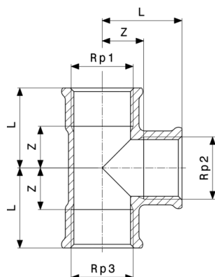
T-kus - mosadz model 1622
