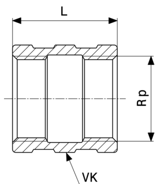
Spojka - červený bronz alebo kremíkový bronz model 3270
