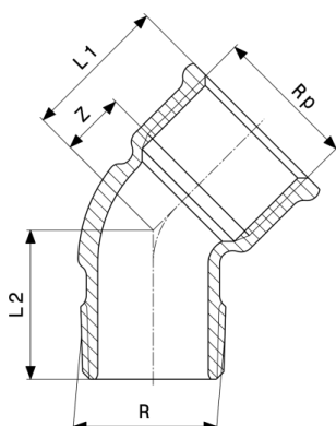
Oblúk 45° - červený bronz alebo kremíkový bronz model 3121
