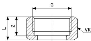
Prevlečná matica - mosadz model 1121-654
