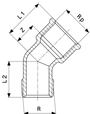
Oblúk 45° - mosadz model 1615
