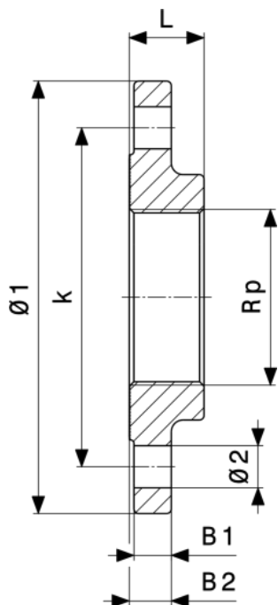
Sanpress XL-príruba - červený bronz alebo kremíkový bronz model 2259.2XL
