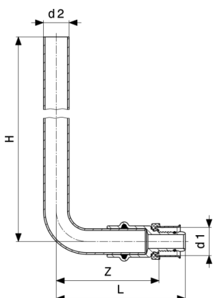
Pexfit Pro-súprava pripojovacieho oblúka model 4777
