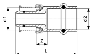
Pexfit Pro-prechodový kus - červený bronz model 4713P
