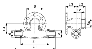
Pexfit Pro-nástenka T-kus - červený bronz model 4724.3
