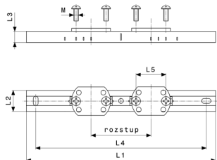
Držiak - ocel pozinkovaná model 2141.3
