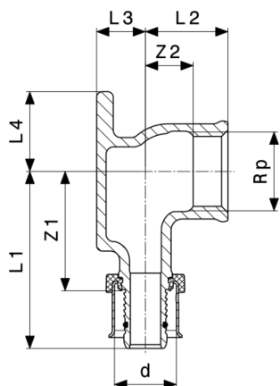
Pexfit Pro-nástenka - červený bronz model 4725.5
