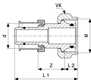
Pexfit Pro-pripájací skrutkový spoj - červený bronz model 4783
