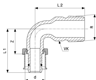
Pexfit Pro-prechodový oblúk 90° - červený bronz model 4714
