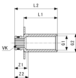
Stenová priechodka model 2032.1
