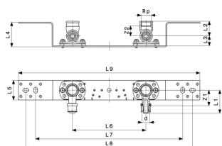
Pexfit Pro-montážna jednotka - ocel' pozinkovaná model 4721.71
