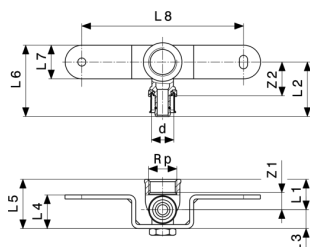
Pexfit Pro-montážna jednotka model 4723
