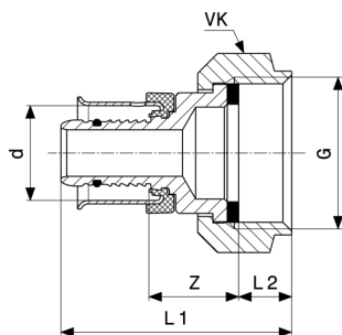
Pexfit Pro-připájecí škrutkový spoj - červený bronz model 4763
