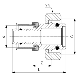
Pexfit Pro-připájecí skrutkový spoj - červený bronz model 4722P
