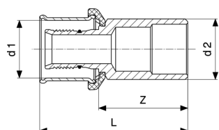
Pexfit Pro-zásuvný kus - červený bronz model 2713
