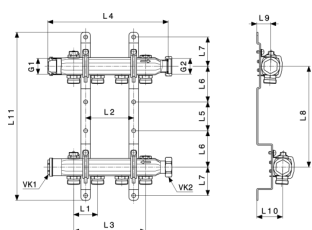
Rozdelovač - ušľachtilá oceľ model 1078
