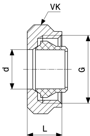
Pripájací skrutkový spoj - mosadz poniklovaná model 94385.2
