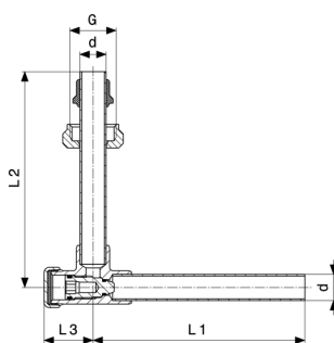
Pripojovacia súprava k vykurovaciemu telesu - mosadz poniklovaná model 2272.5
