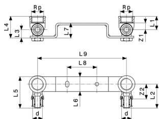
Pexfit Pro-montážna jednotka - červený bronz model 4724
