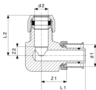
Pexfit Pro-pripojovacie koleno 90° - červený bronz model 4714.7
