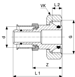
Pexfit Pro-připájecí skrutkový spoj - červený bronz model 4735
