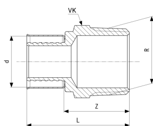
Pexfit Pro-prechodový kus - červený bronz model 2711
