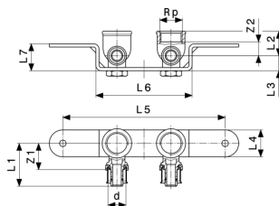
Pexfit Pro-montážna jednotka model 4723.1
