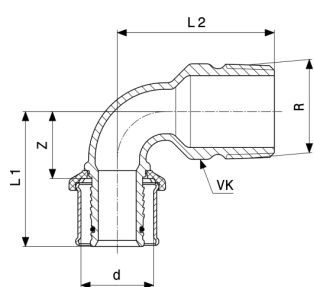
Pexfit Pro-prechodový oblúk 90° - červený bronz model 2714
