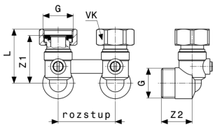
Pripojovací kus k vykurovaciemu telesu - mosadz matne poniklovaná model 1097.5
