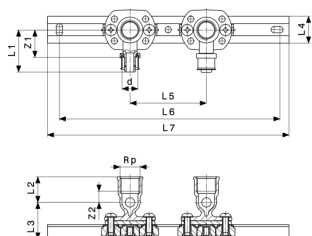
Pexfit Pro-montážna jednotka - ocel' pozinkovaná model 4741
