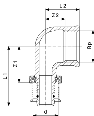
Pexfit Pro-prechodový oblúk 90° - červený bronz model 4714.1
