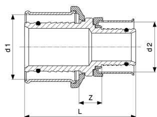
Pexfit Pro-spojka - červený bronz model 4715.7
