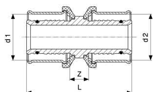
Pexfit Pro-spojka - červený bronz model 2715
