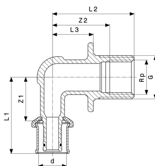
Pexfit Pro-stenová priechodka - červený bronz model 4732.11
