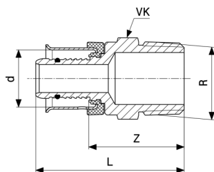
Pexfit Pro-prechodový kus - červený bronz model 4711
