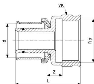
Pexfit Pro-prechodový kus - červený bronz model 2712
