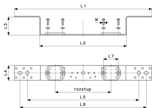
Držiak - oceľ pozinkovaná model 2021.7
