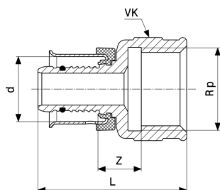
Pexfit Pro-prechodový kus - červený bronz model 4712
