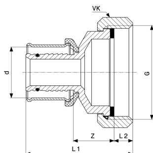
Pexfit Pro-připájecí škrutkový spoj - červený bronz model 2763
