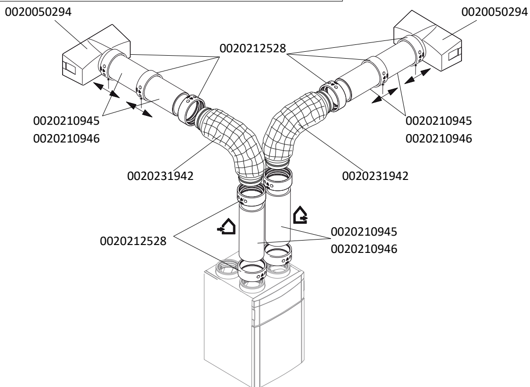
Príklad pripojenia rekuperačnej jednotky k rozdeľovačom vzduchu.
