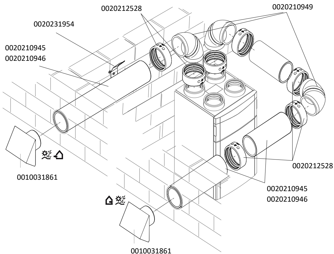
Príklad pripojenia rekuperačnej jednotky k rozdeľovačom vzduchu.
