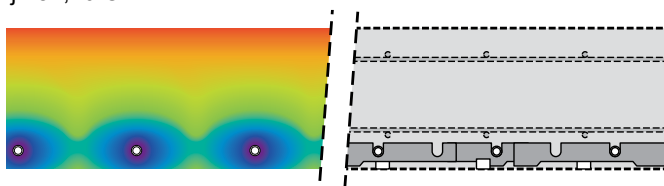
Uponor Contec ON s rozstupom rúrok 170 mm.
