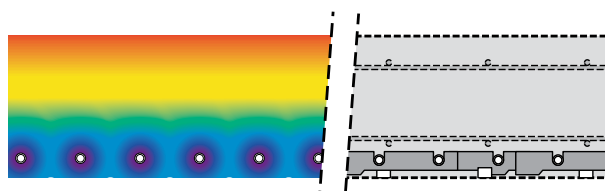
Uponor Contec ON s rozstupom rúrok 85 mm.
