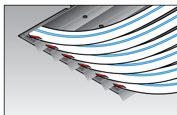
Potrubie so stropným prechodovým prvkom Uponor Contec pre pripojenie do rozdeľovača umiestnenom pod stropom. Smer priebehu je zobrazený červenou styčnicou v stropnom prechodovom prvku.
