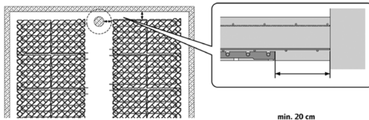
Minimálna vzdialenosť systémovej dosky od vertikálnych nosných konštrukcií.
