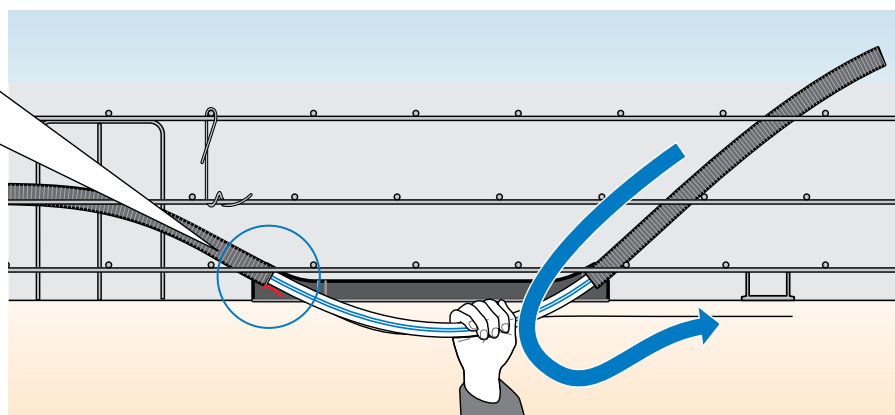
Potrubie so stropným prechodovým prvkom Uponor Contec pre pripojenie do rozdeľovača umiestnenom pod stropom. Smer priebehu je zobrazený červenou styčnicou v stropnom prechodovom prvku.
