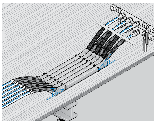
Uponor stropné prechodové prvky na debnení a tlaková skúška pripojovacích potrubí.
