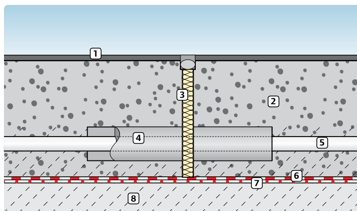
Schéma dilatačnej škáry
